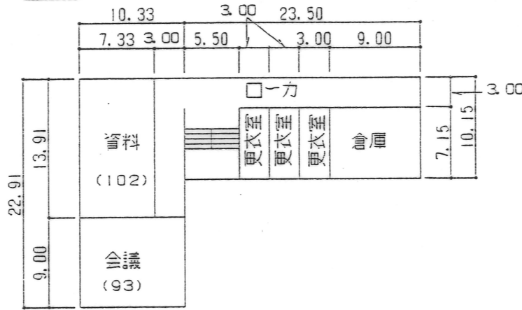
地階
