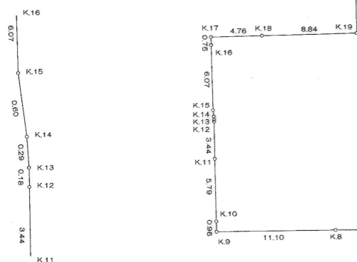
拡大図 S=1:25
